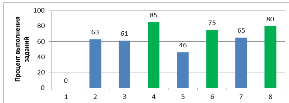
Рис. 3 Качество выполнения тестовых заданий.
