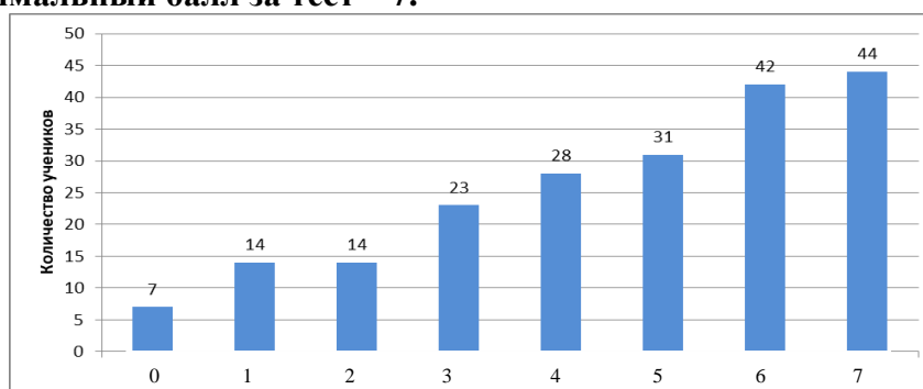
Рис. 2 Выполнение тестовых заданий
